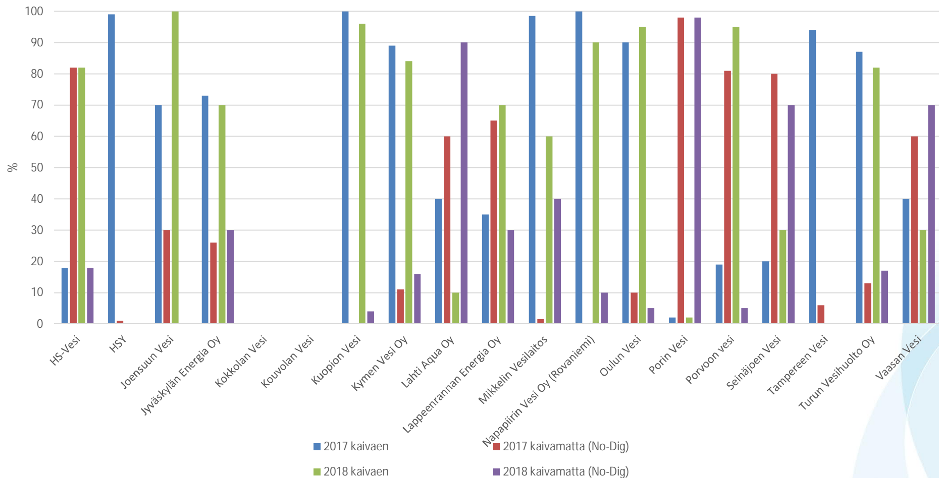
Vesijohtoverkoston saneerausmenetelmät vuosina 2017 ja 2018
